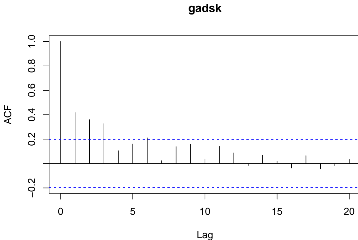
Att. 9.3: Priedu gadskārtu platumu autokorelācijas attēls
